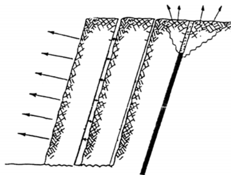
شکل ۶-۱۶- پرتاب سنگ در نتیجه تاخیر کم در آزادسازی مطلوب ردیف‌ها
