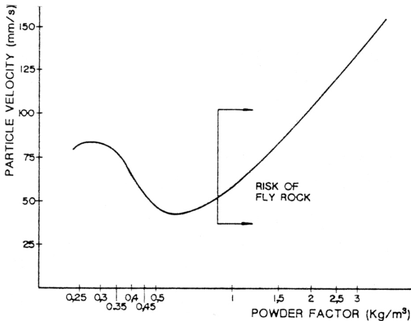
شکل ۸-۶- تاثیر خرج ویژه بر شدت لرزش
